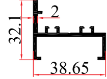
KALIP NO MOLD NUMBER رقم القالب 1332 AĞIRLIK WEIGHT الوزن 0,499 kg/mt
