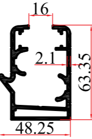
KALIP NO MOLD NUMBER رقم القالب 3762 AĞIRLIK WEIGHT الوزن 1,520 kg/mt
