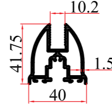
KALIP NO MOLD NUMBER رقم القالب 3899 AĞIRLIK WEIGHT الوزن 0,929 kg/mt
