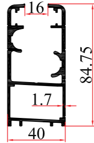
KALIP NO MOLD NUMBER رقم القالب 3901 AĞIRLIK WEIGHT الوزن 1,746 kg/mt
