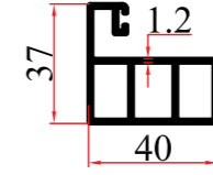
KALIP NO MOLD NUMBER رقم القالب 3876 AĞIRLIK WEIGHT الوزن 0,623 kg/mt
