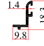
KALIP NO MOLD NUMBER رقم القالب 382 AĞIRLIK WEIGHT الوزن 0,170 kg/mt
