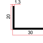
KALIP NO MOLD NUMBER رقم القالب 10114 AĞIRLIK WEIGHT الوزن 0,171 kg/mt
