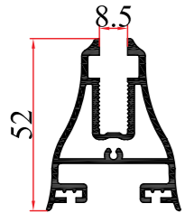
KALIP NO MOLD NUMBER رقم القالب 2134 AĞIRLIK WEIGHT الوزن 1,069 kg/mt
