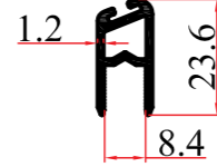
KALIP NO MOLD NUMBER رقم القالب 3807 AĞIRLIK WEIGHT الوزن 0,224 kg/mt
