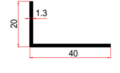
KALIP NO MOLD NUMBER رقم القالب 17 AĞIRLIK WEIGHT الوزن 0,206 kg/mt
