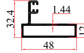
KALIP NO MOLD NUMBER رقم القالب 3764 AĞIRLIK WEIGHT الوزن 0,435 kg/mt
