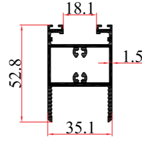
KALIP NO MOLD NUMBER رقم القالب 1333 AĞIRLIK WEIGHT الوزن 1,034 kg/mt
