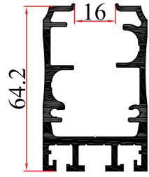
KALIP NO MOLD NUMBER رقم القالب 2140 AĞIRLIK WEIGHT الوزن 1,717 kg/mt
