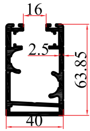
KALIP NO MOLD NUMBER رقم القالب 3975 AĞIRLIK WEIGHT الوزن 1,680 kg/mt
