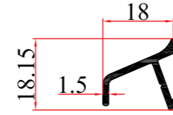
KALIP NO MOLD NUMBER رقم القالب 3980 AĞIRLIK WEIGHT الوزن 0,119 kg/mt
