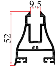
KALIP NO MOLD NUMBER رقم القالب 2131 AĞIRLIK WEIGHT الوزن 1,029 kg/mt
