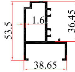
KALIP NO MOLD NUMBER رقم القالب 1331 AĞIRLIK WEIGHT الوزن 0,848 kg/mt
