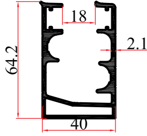
KALIP NO MOLD NUMBER رقم القالب 1320 AĞIRLIK WEIGHT الوزن 1,409 kg/mt
