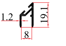
KALIP NO MOLD NUMBER رقم القالب 3775 AĞIRLIK WEIGHT الوزن 0,141 kg/mt
