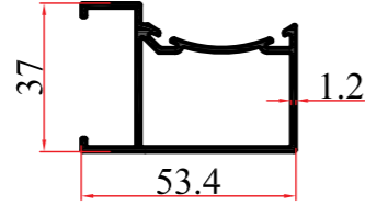
KALIP NO MOLD NUMBER رقم القالب 1326 AĞIRLIK WEIGHT الوزن 0,621 kg/mt
