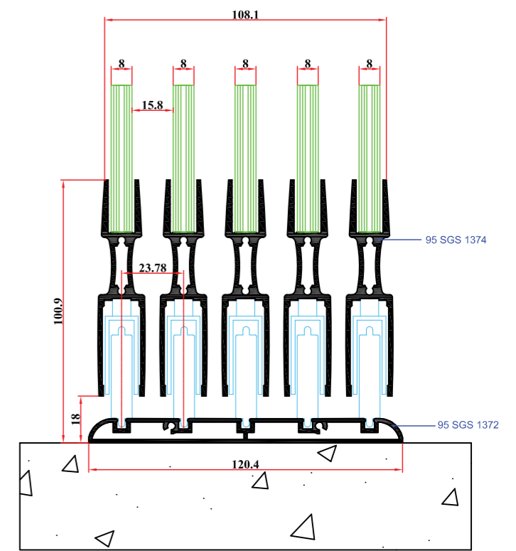
2a NOLU DETAY ÖLÇEK:1/2
