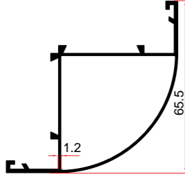
KALIP NO MOLD NUMBER رقم القالب 167 AĞIRLIK WEIGHT الوزن 0,752 kg/mt
