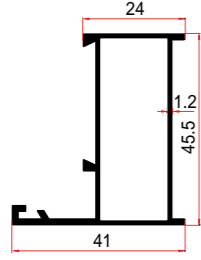
KALIP NO MOLD NUMBER رقم القالب 150 AĞIRLIK WEIGHT الوزن 0,535 kg/mt
