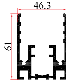
KALIP NO MOLD NUMBER رقم القالب 2138 AĞIRLIK WEIGHT الوزن 1,785 kg/mt
