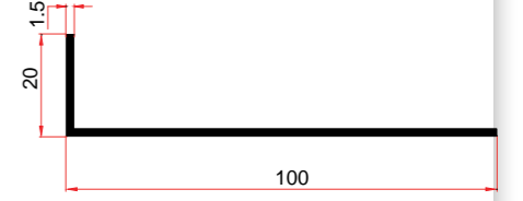
KALIP NO MOLD NUMBER رقم القالب 10130 AĞIRLIK WEIGHT الوزن 0,480 kg/mt
