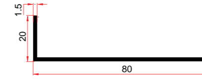
KALIP NO MOLD NUMBER رقم القالب 10129 AĞIRLIK WEIGHT الوزن 0,399 kg/mt
