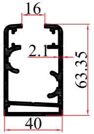
KALIP NO MOLD NUMBER رقم القالب 3761 AĞIRLIK WEIGHT الوزن 1,460 kg/mt
