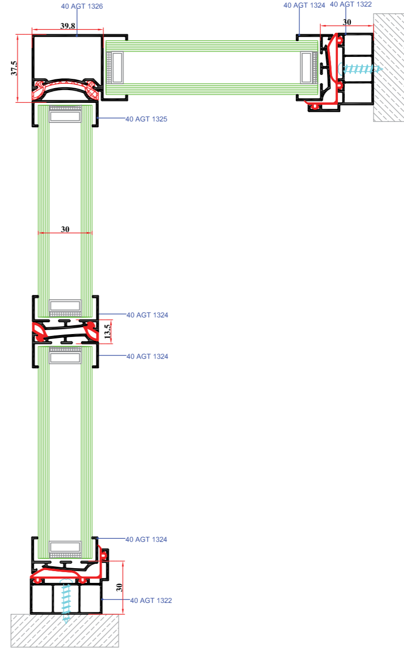
1 NOLU DETAY ÖLÇEK:1/2
