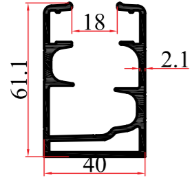
KALIP NO MOLD NUMBER رقم القالب 1330 AĞIRLIK WEIGHT الوزن 1,366 kg/mt
