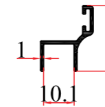
KALIP NO MOLD NUMBER رقم القالب 3983 AĞIRLIK WEIGHT الوزن 0,146 kg/mt
