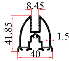
KALIP NO MOLD NUMBER رقم القالب 3763 AĞIRLIK WEIGHT الوزن 0,916 kg/mt
