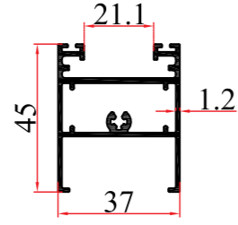
KALIP NO MOLD NUMBER رقم القالب 1321 AĞIRLIK WEIGHT الوزن 0,766 kg/mt
