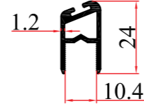
KALIP NO MOLD NUMBER رقم القالب 3985 AĞIRLIK WEIGHT الوزن 0,254 kg/mt
