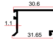
KALIP NO MOLD NUMBER رقم القالب 159 AĞIRLIK WEIGHT الوزن 0,235 kg/mt
