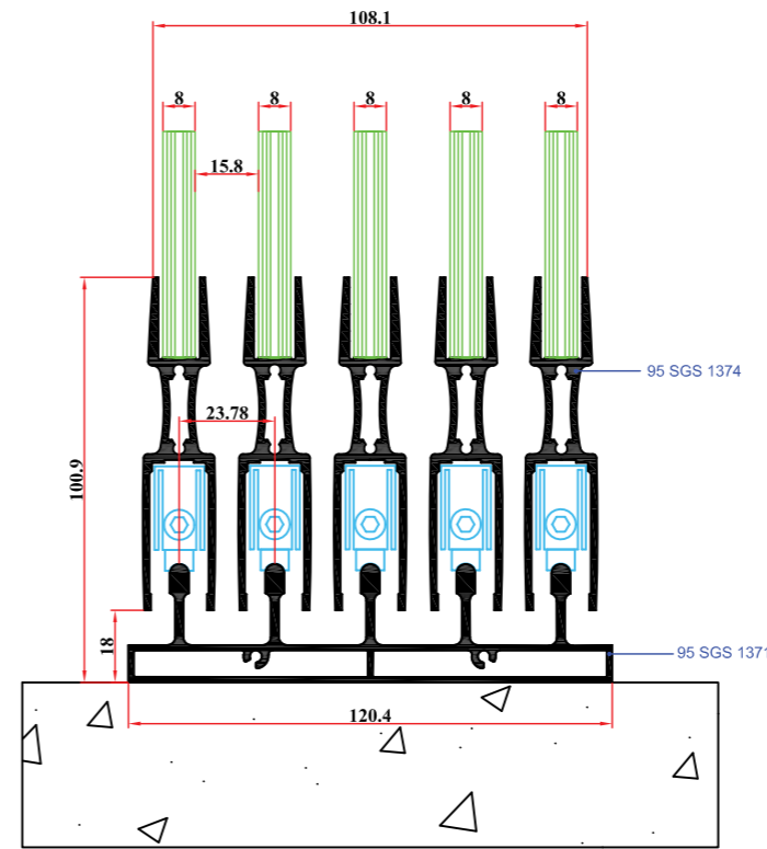
2 NOLU DETAY ÖLÇEK:1/2
