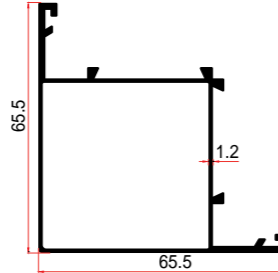
KALIP NO MOLD NUMBER رقم القالب 182 AĞIRLIK WEIGHT الوزن 0,814 kg/mt
