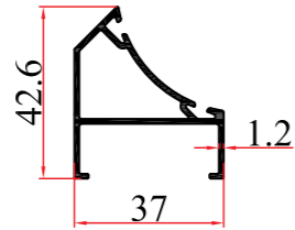
KALIP NO MOLD NUMBER رقم القالب 1328 AĞIRLIK WEIGHT الوزن 0,475 kg/mt
