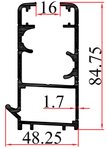
KALIP NO MOLD NUMBER رقم القالب 3900 AĞIRLIK WEIGHT الوزن 1,824 kg/mt
