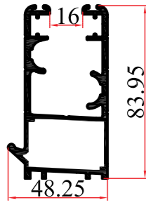
KALIP NO MOLD NUMBER رقم القالب 3974 AĞIRLIK WEIGHT الوزن 1,799 kg/mt
