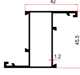
KALIP NO MOLD NUMBER رقم القالب 151 AĞIRLIK WEIGHT الوزن 0,642 kg/mt
