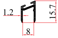
KALIP NO MOLD NUMBER رقم القالب 3776 AĞIRLIK WEIGHT الوزن 0,126 kg/mt
