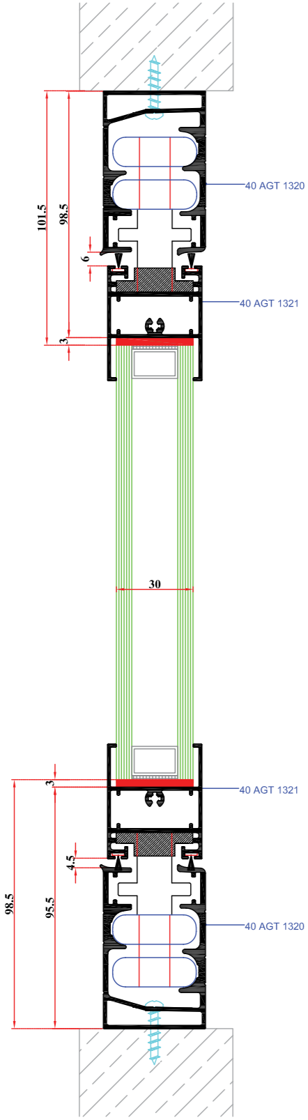
1 NOLU DETAY TOPLAM CAM BOŞLUĞU 98.5+101.5 = 200 mm'dir
