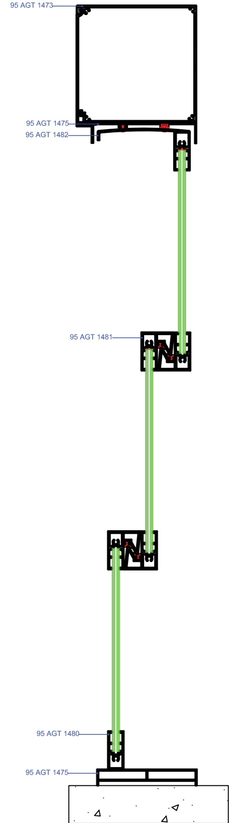
2 NOLU DETAY
