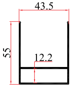
KALIP NO MOLD NUMBER رقم القالب 2143 AĞIRLIK WEIGHT الوزن 0,680 kg/mt
