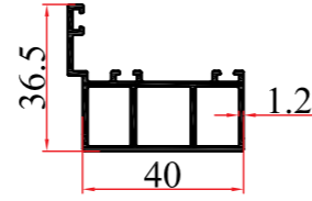
KALIP NO MOLD NUMBER رقم القالب 1322 AĞIRLIK WEIGHT الوزن 0,594 kg/mt
