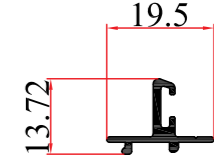
KALIP NO MOLD NUMBER رقم القالب 2133 AĞIRLIK WEIGHT الوزن 0,132 kg/mt
