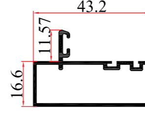
KALIP NO MOLD NUMBER رقم القالب 2144 AĞIRLIK WEIGHT الوزن 0,445 kg/mt
