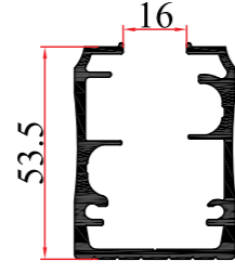
KALIP NO MOLD NUMBER رقم القالب 2130 AĞIRLIK WEIGHT الوزن 1,314 kg/mt
