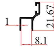
KALIP NO MOLD NUMBER رقم القالب 3766 AĞIRLIK WEIGHT الوزن 0,140 kg/mt
