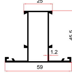
KALIP NO MOLD NUMBER رقم القالب 152 AĞIRLIK WEIGHT الوزن 0,642 kg/mt
