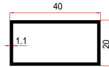
KALIP NO MOLD NUMBER رقم القالب 10 AĞIRLIK WEIGHT الوزن 0,343 kg/mt
