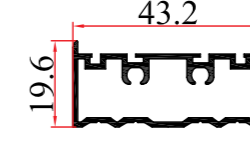
KALIP NO MOLD NUMBER رقم القالب 2132 AĞIRLIK WEIGHT الوزن 0,478 kg/mt
