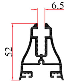
KALIP NO MOLD NUMBER رقم القالب 2135 AĞIRLIK WEIGHT الوزن 1,118 kg/mt
