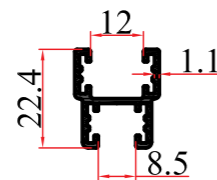
KALIP NO MOLD NUMBER رقم القالب 3877 AĞIRLIK WEIGHT الوزن 0,260 kg/mt
