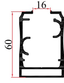
KALIP NO MOLD NUMBER رقم القالب 2145 AĞIRLIK WEIGHT الوزن 1,363 kg/mt
