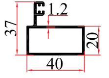
KALIP NO MOLD NUMBER رقم القالب 3788 AĞIRLIK WEIGHT الوزن 0,498 kg/mt
