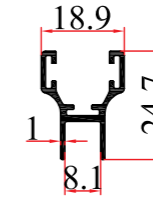
KALIP NO MOLD NUMBER رقم القالب 3765 AĞIRLIK WEIGHT الوزن 0,226 kg/mt
