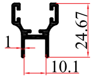
KALIP NO MOLD NUMBER رقم القالب 3982 AĞIRLIK WEIGHT الوزن 0,246 kg/mt
