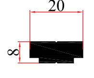
KALIP NO MOLD NUMBER رقم القالب 2139 AĞIRLIK WEIGHT الوزن 0,394 kg/mt
