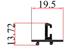
KALIP NO MOLD NUMBER رقم القالب 2133 AĞIRLIK WEIGHT الوزن 0,132 kg/mt
