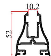
KALIP NO MOLD NUMBER رقم القالب 2141 AĞIRLIK WEIGHT الوزن 1,131 kg/mt
