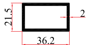
KALIP NO MOLD NUMBER رقم القالب 3902 AĞIRLIK WEIGHT الوزن 0,580 kg/mt
