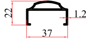
KALIP NO MOLD NUMBER رقم القالب 1325 AĞIRLIK WEIGHT الوزن 0,338 kg/mt
