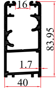
KALIP NO MOLD NUMBER رقم القالب 3973 AĞIRLIK WEIGHT الوزن 1,723 kg/mt
