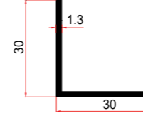
KALIP NO MOLD NUMBER رقم القالب 28 AĞIRLIK WEIGHT الوزن 0,205 kg/mt
