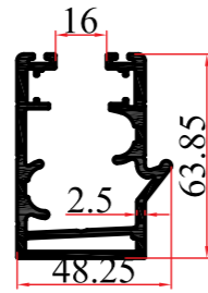
KALIP NO MOLD NUMBER رقم القالب 3976 AĞIRLIK WEIGHT الوزن 1,741 kg/mt
