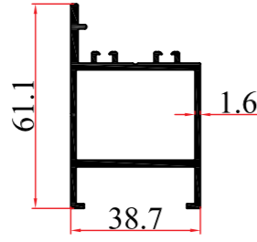
KALIP NO MOLD NUMBER رقم القالب 1334 AĞIRLIK WEIGHT الوزن 0,942 kg/mt
